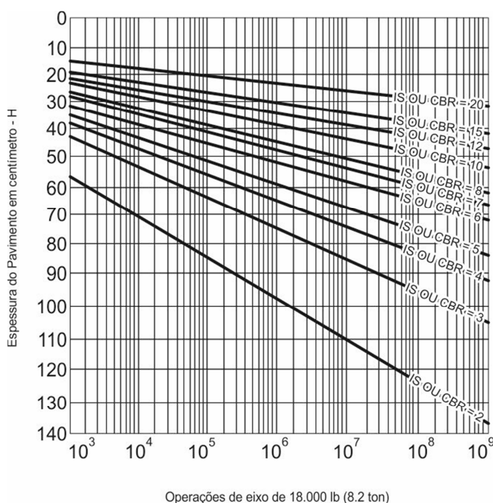
Espessura do Pavimento em Termos de Base Granular ( K = 1 ) em Função de N
