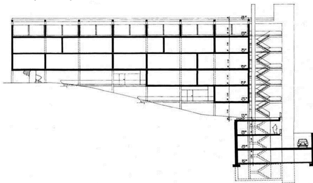
Corte pelas unidades
