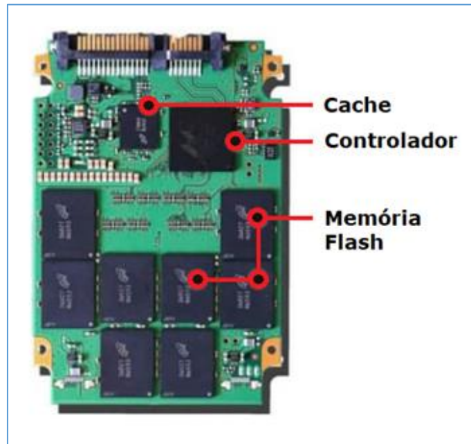
Figura 5 – Placa de circuito de dispositivo de armazenamento
