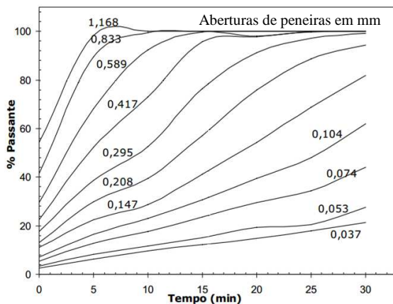
Figura 1 - Curva de moagem do minério de feldspato pegmatítico
