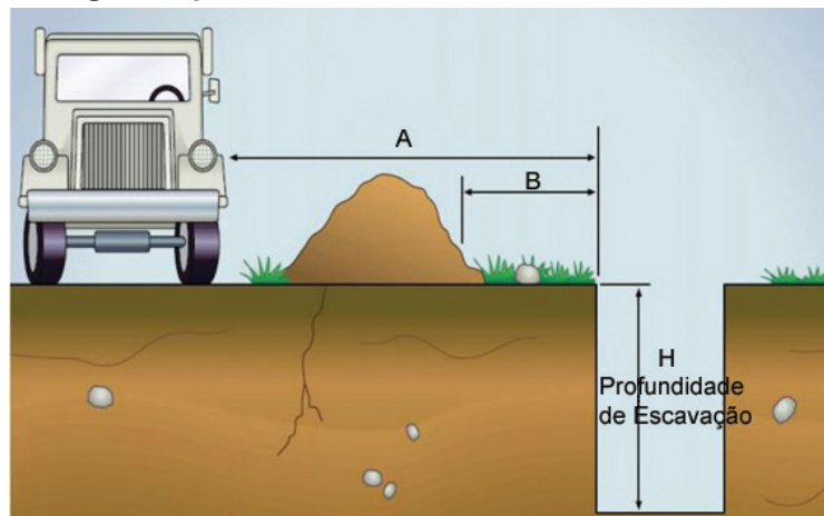
Figura 1 - Medidas de afastamento mínimo.
