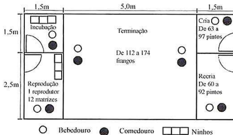
Planta baixa das instalações para o sistema alternativo de criação de galinhas caipiras.
