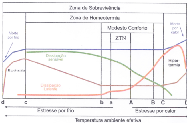
Representação esquemática das temperaturas ambientais efetivas. Adaptado de Sallvik (1999).
